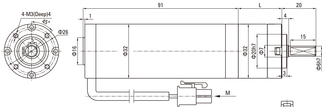
外径32ブラシレス遊星減速モーターの外観図
