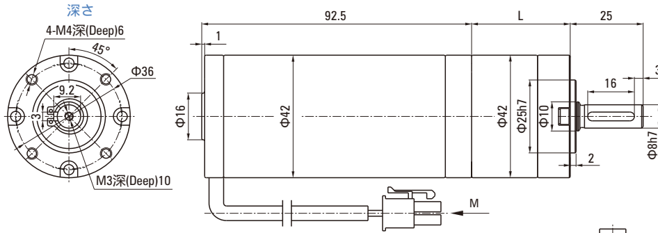
M方向から見る M向视图 (View M)
