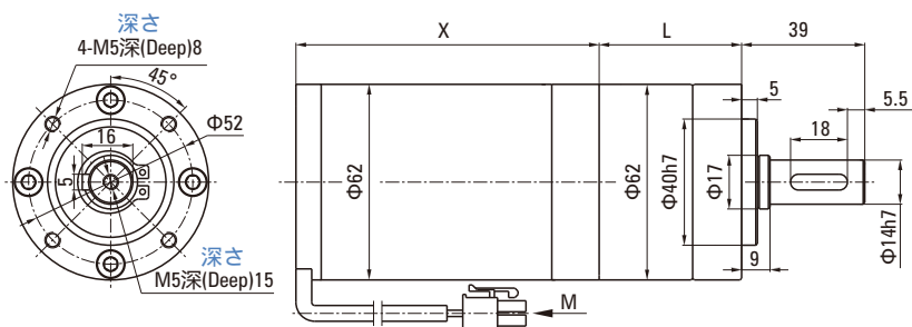
M方向から見る M向视图 (View M)
